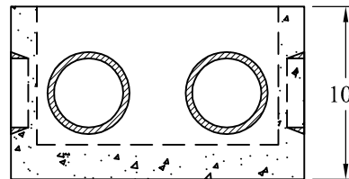
Outlet End
