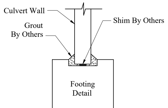
Typ Footings
