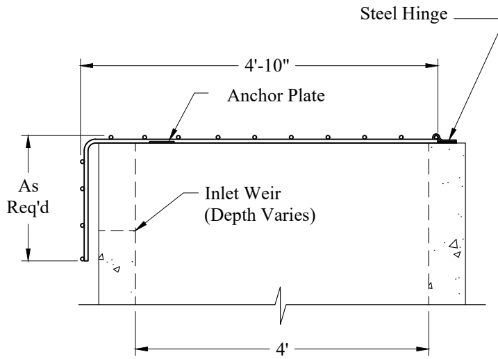
Side View Typ 4' x 4' OCS
