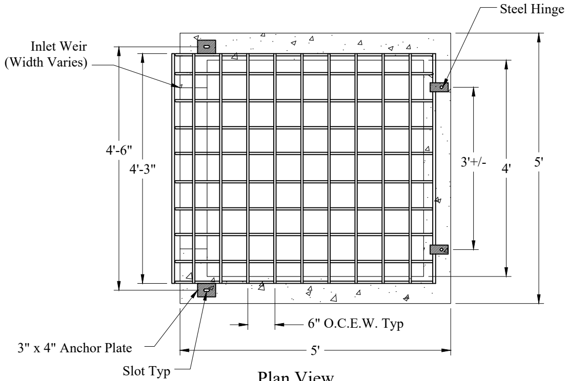
Plan View Typ 4' x 4' OCS
